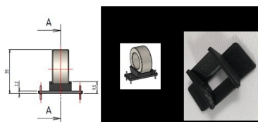
Exemple d'embases
